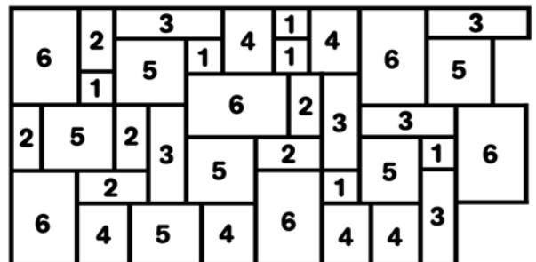
SKLADBA OBKLADU NA VÝŠKU 102 cm
