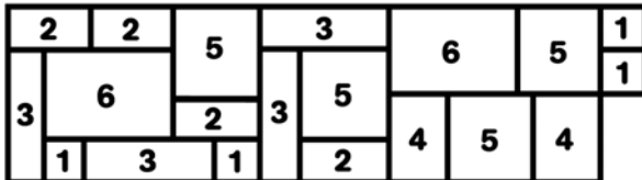
SKLADBA OBKLADU NA VÝŠKU 50 cm
